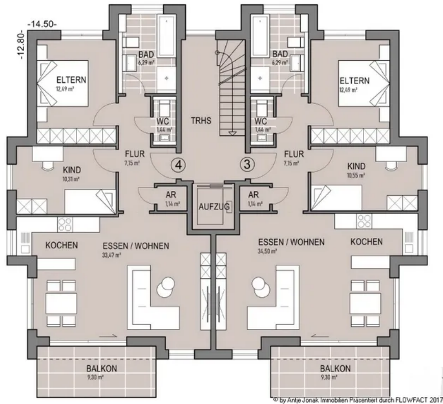
Obergeschoss
