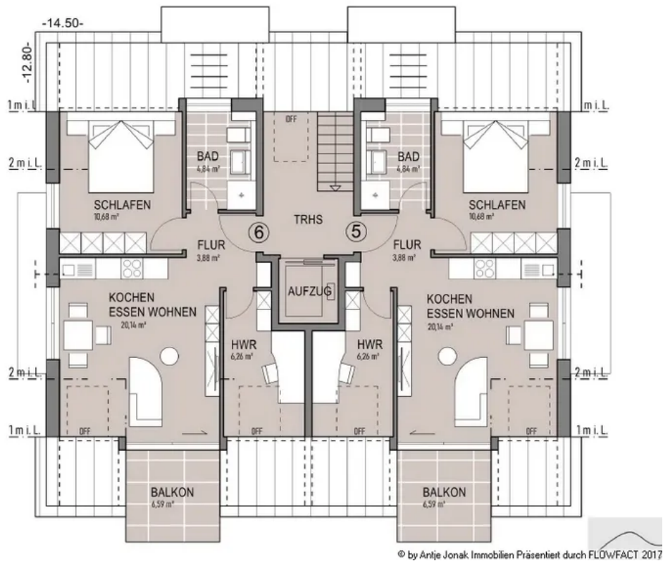
Dachgeschoss
